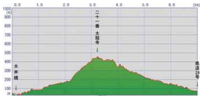
二十一番 太龍寺 縦断図
